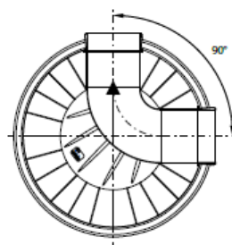
Fond profilé coude 90°
